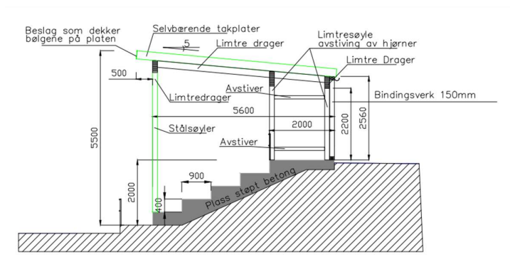
SNITT AA
